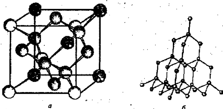
Р и с . 4.7. Структура алмаза: а – решетка; б – схема направлений химических связей
