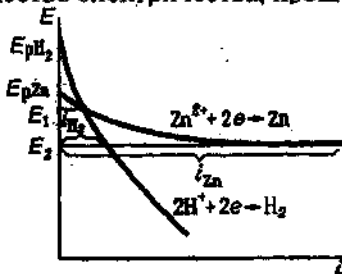
Рис. 9.12. Поляризационные кривые катодного выделения водорода и цинка
