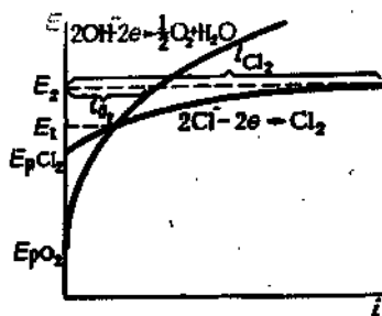
Рис. 9.13. Поларизационные кривые анодного выделения кислорода и хлора
