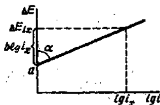
Рис. 9.10. Зависимости электрохимической поляризации электродов от \lg i
