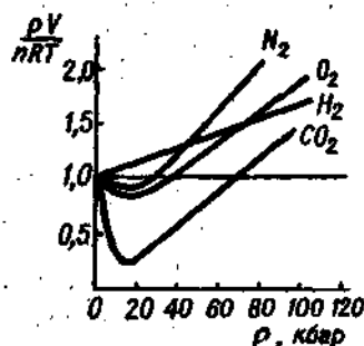
Рис. 4.3. Отклонение свойств реальных газов от свойств идеальных газов при температуре 273 K
