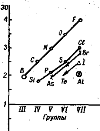
Рис. 12.3. Изменение электроотрицательности неметаллов по периодам
