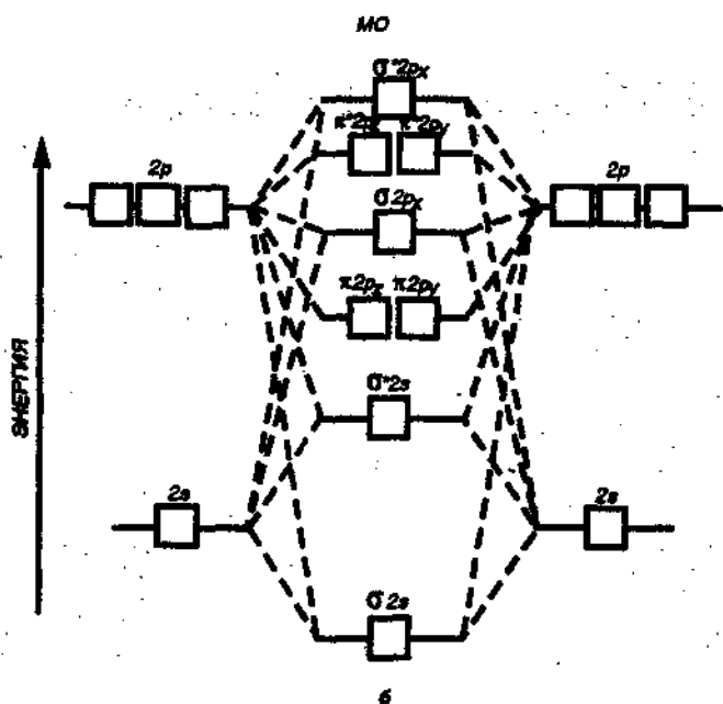
Р и с . 2.16. Диаграмма энергетических уровней АО и МО двухатомных молекул элементов от начала (до N_2 ) (а) и до конца (от N_2 до F_2 ) (б) второго периода
