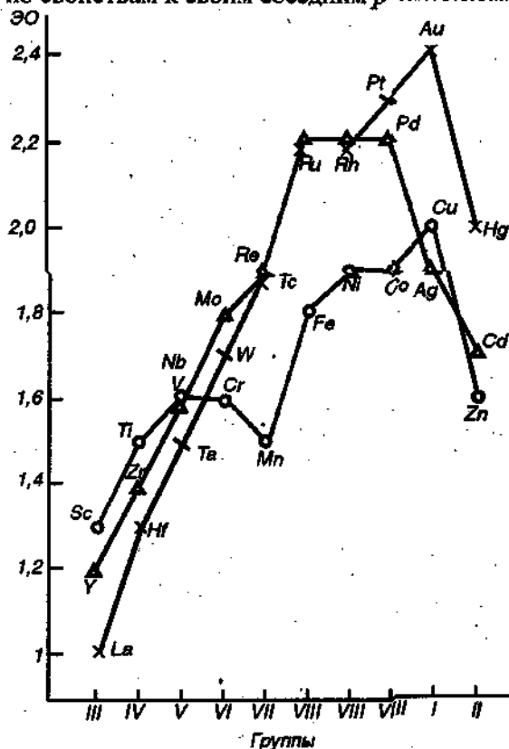
Рис. 11.12. Изменение электроотрицательности d -элементов по группам
