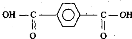
терефталевая кислота
