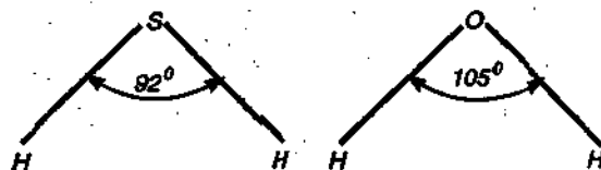
Рис. 2.10. Валентные углы у молекул \text{H}_2\text{S} , \text{H}_2\text{O}
