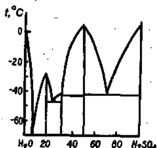
Рис. 6.6. Диаграмма плавкости системы \text{H}_2\text{O}-\text{H}_2\text{SO}_4
