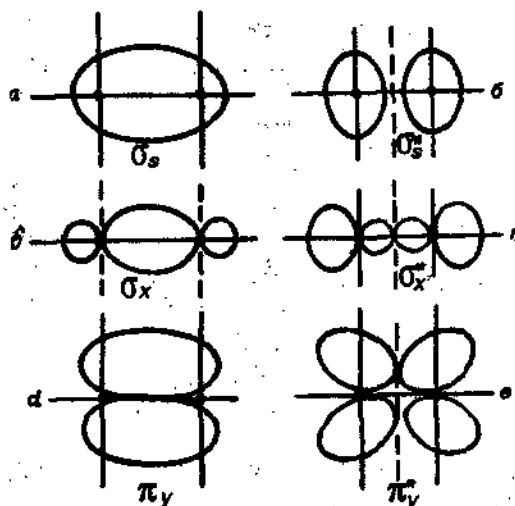
Рис. 2.14. Контуры формы связывающих (а, в, д) и разрыхляющих (б, з, е) МО, образованных при перекрывании s(a, b) , p_x(a, z) и p_y(d, e) -АО
