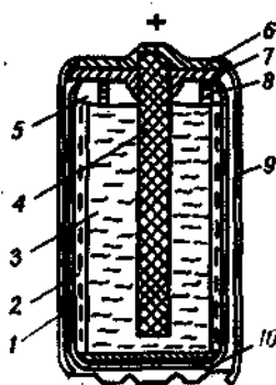
Рис. 9.15. Схема первичного элемента \text{MnO}_2 — \text{Zn} с соевым электролитом:
