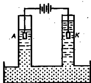
Рис. 8.8. Схема устройства для демонстрации электрофореза
