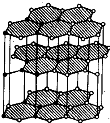
Рис. 4.9. Структура графита
