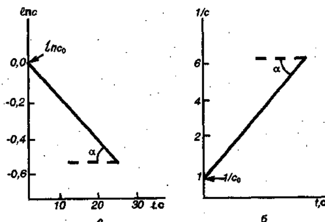
Рис. 7.1. Изменение концентраций исходных веществ во времени для реакций первого (а) и второго (б) порядков
