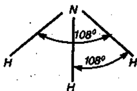
Рис. 2.11. Валентные углы у молекулы \text{NH}_3
