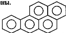
Бенз(а)пирен (БП)
