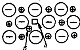
Рис. 4.13. Точечный дефект в ионном кристалле в узле решетки (а) при перемещении иона в междоузлие (б)
