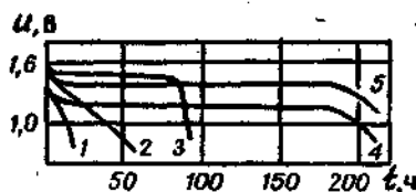
Рис. 9.16. Разрядные кривые первичных элементов одинаковой массы: марганцево-цинковых с соевым (1) и щелочным (2) электролитом, серебряно-цинкового (3), воздушно-цинкового (4) и сульфиджелезно-литиевого с неводным раствором электролита (5)
